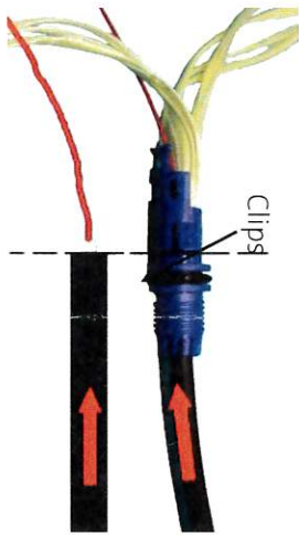
2 Push the cable up to the clips / Pousser le câble jusqu'aux clips
